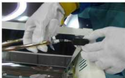
4. DESENFILER DE LA LAMPE LES DEUX JOINTS SILICONIQUES ET DECONNECTER LES DEUX FASTONS QUI FONT LA CONNECTION ELECTRIQUE
